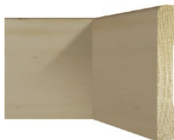
PENCIL ROUND 6mm 1 edge 42 | 68 | 92 x 18
